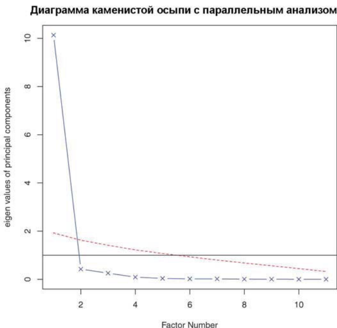
Рис. 14.2. Оценка числа главных компонент, достаточного для характеристики данных из примера про американских судей. График собственных значений (линия с крестиками), критерия превышения собственными значениями единицы (горизонтальная линия) и параллельный анализ со 100 симуляциями (пунктир) свидетельствуют о том, что достаточно использовать одну компоненту
