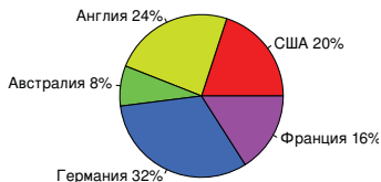
Круговая диаграмма с процентами
