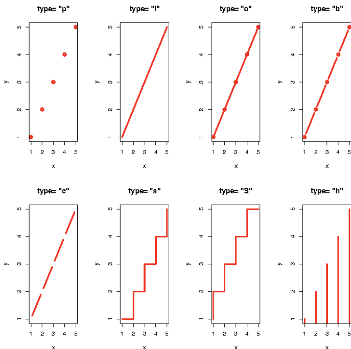
Рис. 11.18. Диаграммы, полученные при разных значениях параметра type функций plot() и lines()
