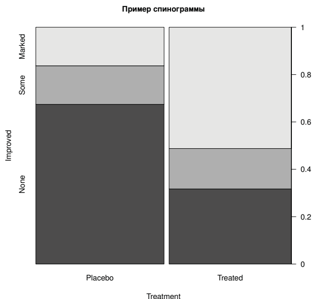
Рис. 6.5. Спинограмма, на которой отражены результаты лечения артрита
