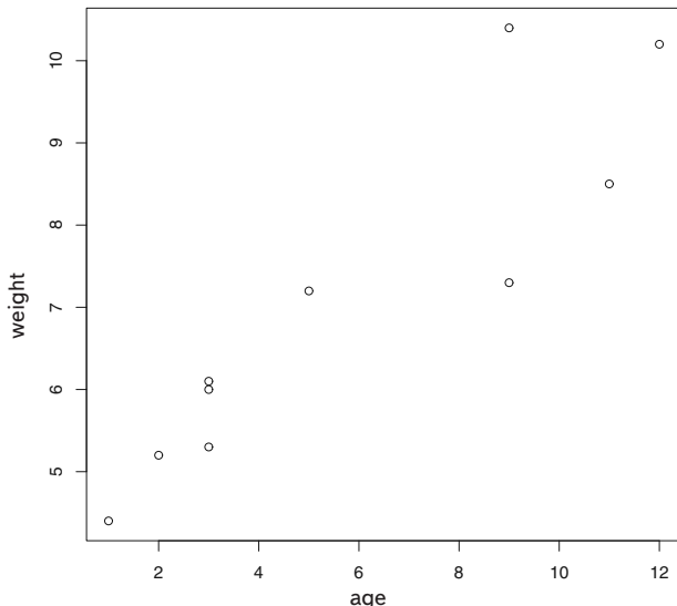
Рис. 1.4. Диаграмма рассеяния веса младенцев (weight, в килограммах) в зависимости от их возраста (age, в месяцах)
