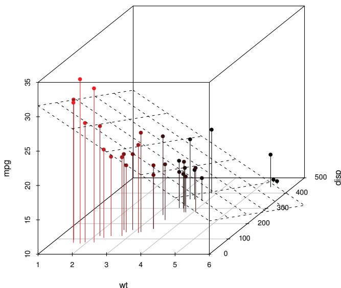
Рис. 11.13. Трехмерная диаграмма рассеяния с вертикальными линиями, градиентом яркости и наложенной регрессионной плоскостью
