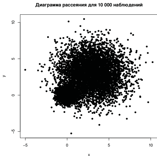
Рис. 11.7. Диаграмма рассеяния для 10 000 наблюдений и с заметным наложением точек друг на друга. Обратите внимание на то, что наложение точек затрудняет обнаружение области с наивысшей их концентрацией
