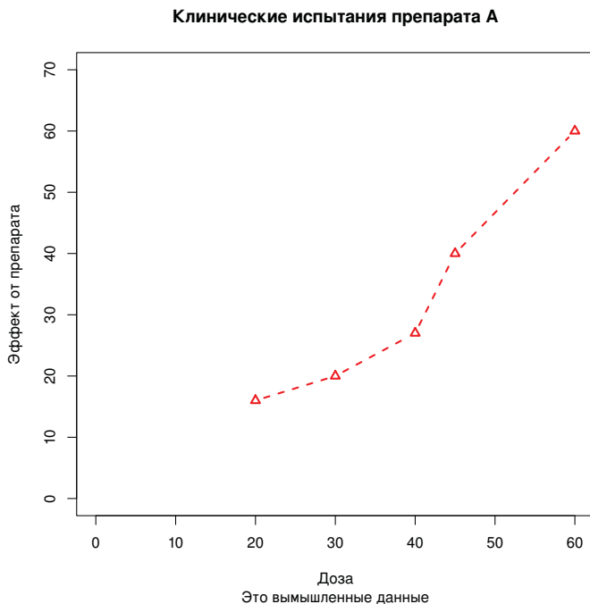
Рис. 3.8. Линейный график зависимости реакции пациента от дозы лекарства А с заголовком, подзаголовком и модифицированными осями
