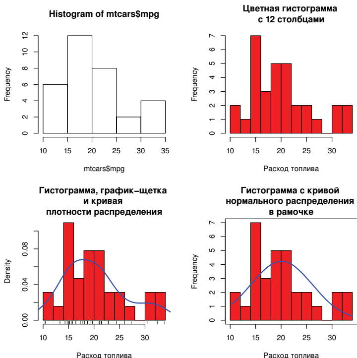
Рис. 6.8. Примеры построения гистограмм
