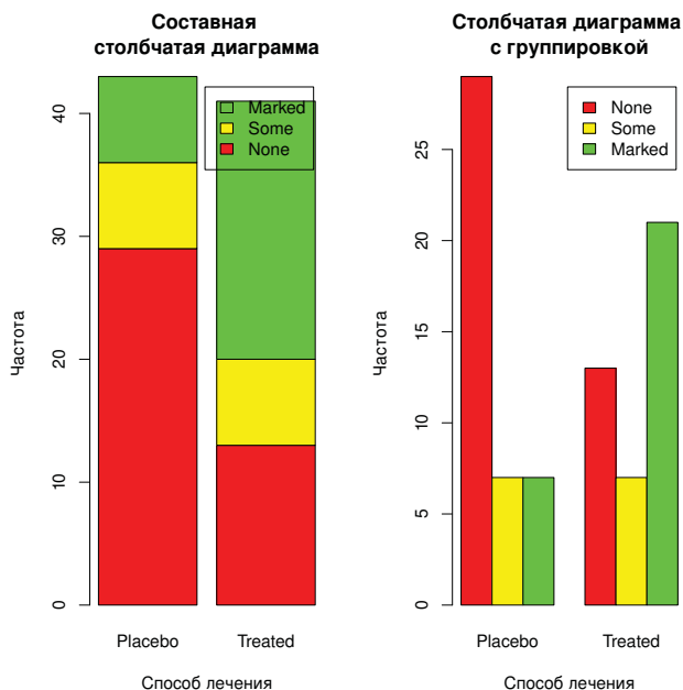
Рис. 6.2. Столбчатые диаграммы: составные и с группировкой
