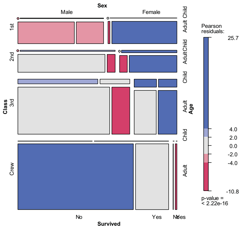
Рис. 11.23. Мозаичная диаграмма, которая характеризует пол, возраст людей, выживших при крушении Титаника, и класс, в котором они путешествовали
