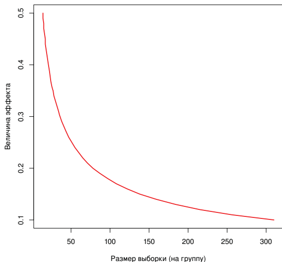
Рис. 10.2. Размеры выборок, необходимые для обнаружения эффектов разной величины при однофакторном дисперсионном анализе с пятью группами (при заданной мощности 0.9 и уровне значимости 0.05)
