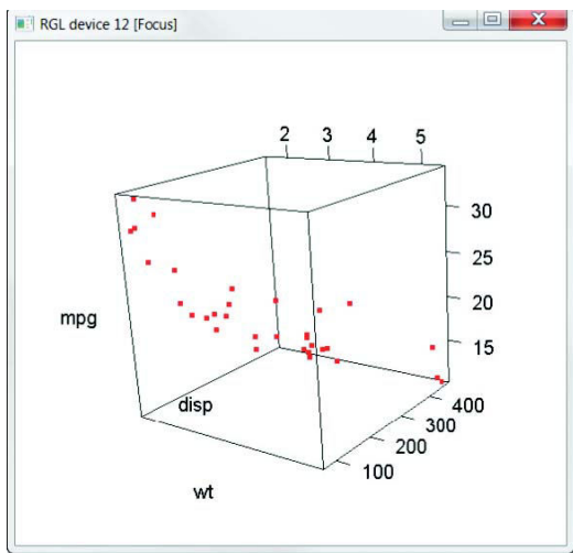
Рис. 11.14. Вращающаяся диаграмма рассеяния, полученная при помощи функции plot3d() из пакета rgl
