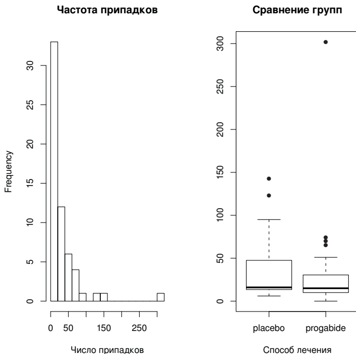
Рис. 13.1. Распределение значений числа припадков после лечения (источник данных: опубликованные данные о припадках (Breslow, 1993))
