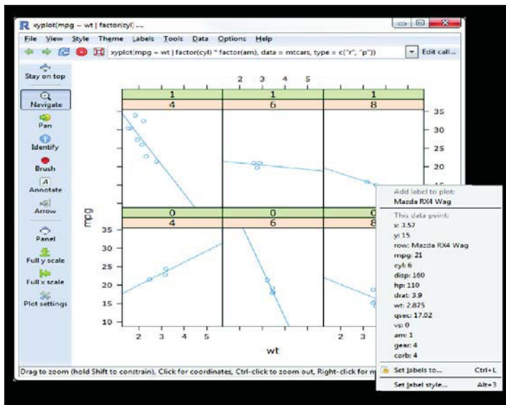
Рис. 16.12. Графический интерфейс GTK+ пакета playwith . В этом интерфейсе пользователь может изменять диаграмму при помощи мыши
