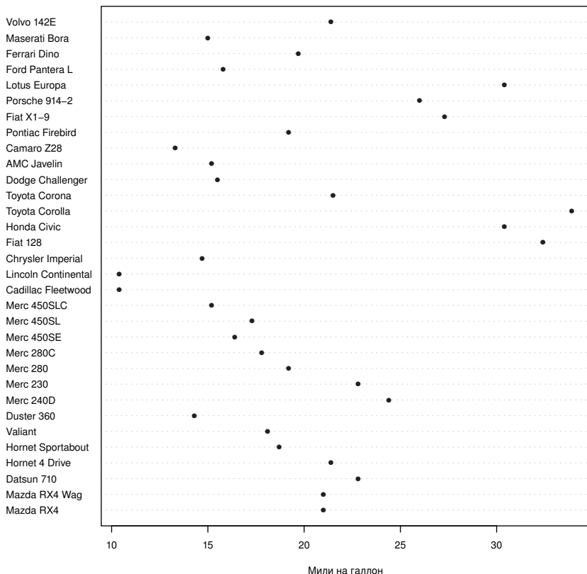
Рис. 6.16. Точечная диаграмма для расхода топлива у автомобилей разных марок
