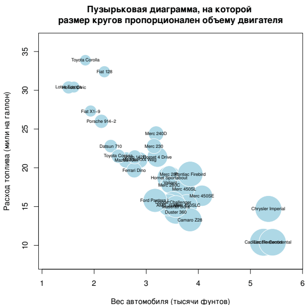
Рис. 11.16. Пузырьковая диаграмма для зависимости между весом автомобиля и расходом топлива, где размер кругов пропорционален объему двигателя
