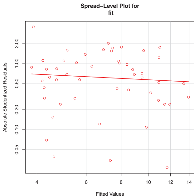
Рис. 8.12. Диаграмма для проверки однородности дисперсии остатков
