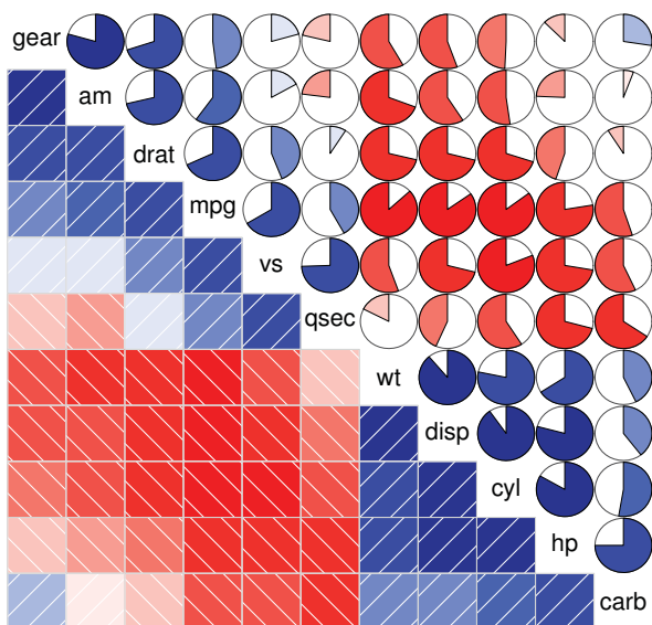
Рис. 11.20. Корреллограмма для корреляций между переменными из таблицы данных mtcars . Порядок строк и столбцов был изменен по результатам анализа главных компонент
