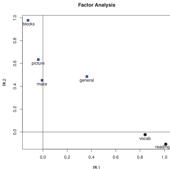
Рис. 14.5. Двухфакторная диаграмма для результатов психологических тестов из набора данных ability.cov . Словарь и чтение сопряжены с первым фактором (FA1), а блоки, картинки и лабиринт – со вторым (FA2). Результаты теста на общее умственное развитие связаны с обоими факторами
