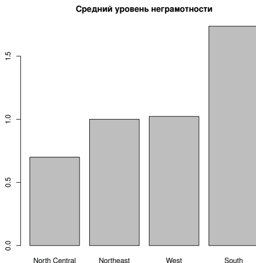
Рис. 6.3. Столбчатая диаграмма для отсортированных в порядке возрастания средних значений неграмотности в разных частях США
