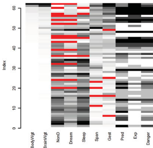
Рис. 15.3. Матричная диаграмма наблюдаемых и пропущенных значений в каждой строке набора данных sleep . Матрица отсортирована по значениям переменной BodyWgt
