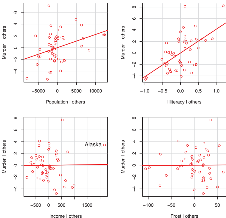
Рис. 8.15. Диаграммы добавленных переменных для исследования вклада влиятельных наблюдений
